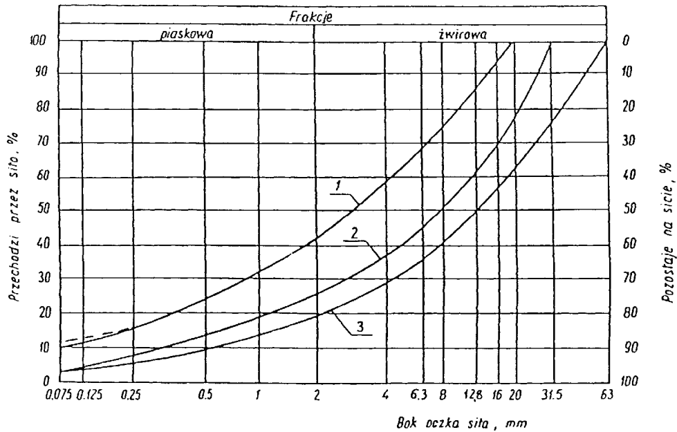
Rysunek 1. Pole dobrego uziarnienia kruszywa przeznaczonych na podbudowy wykonywane metod stabilizacji mechanicznej
