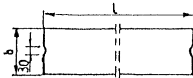
Rys. 1. Wymiarowanie krawników
