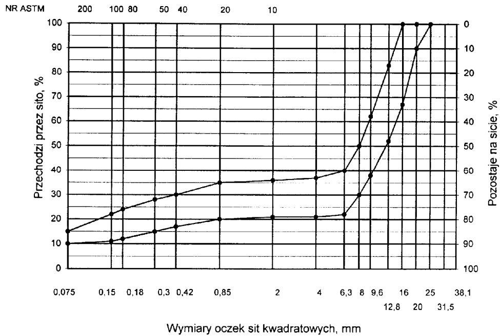
Rys. 5. Krzywe graniczne uziarnienia mieszanki mineralnej BA od 0 do 20 mm (mieszanka o nieci głym uziarnieniu) do warstwy cialnej nawierzchni drogi o obciążeniu ruchem od KR3 do KR6
