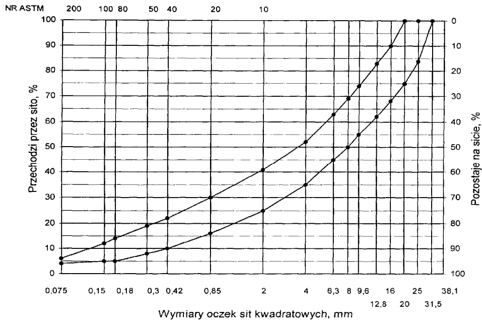
Rys. 12. Krzywe graniczne uziarnienia mieszanki mineralnej BA od 0 do 20 mm do warstwy wiązującej, wyrównawczej i wzmacniającej nawierzchni drogi o obciążeniu ruchem od KR3 do KR6
