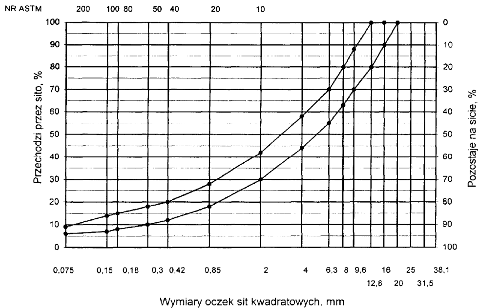
Rys. 5. Krzywe graniczne uziarnienia mieszanki mineralnej BA od 0 do 20 mm (mieszanka o nieci głym uziarnieniu) do warstwy cialnej nawierzchni drogi o obciążeniu ruchem od KR3 do KR6
