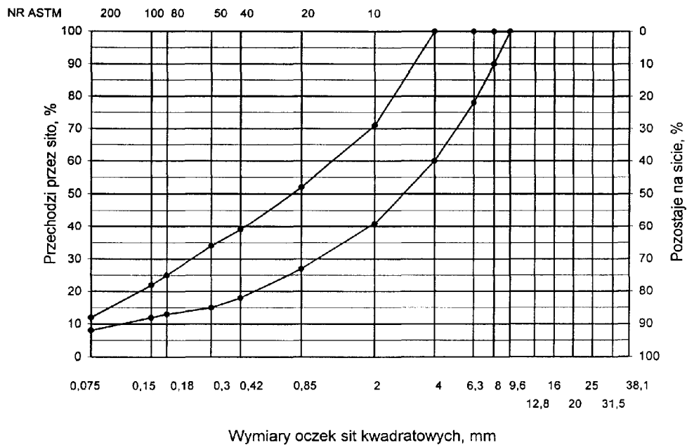
Rys. 3. Krzywe graniczne uziarnienia mieszanki mineralnej BA od 0 do 8mm, od 0 do 6,3 mm do warstwy cieralnej nawierzchni drogi o obciążeniu ruchem nawierzchni drogi o obciążeniu ruchem KR1 lub KR2
