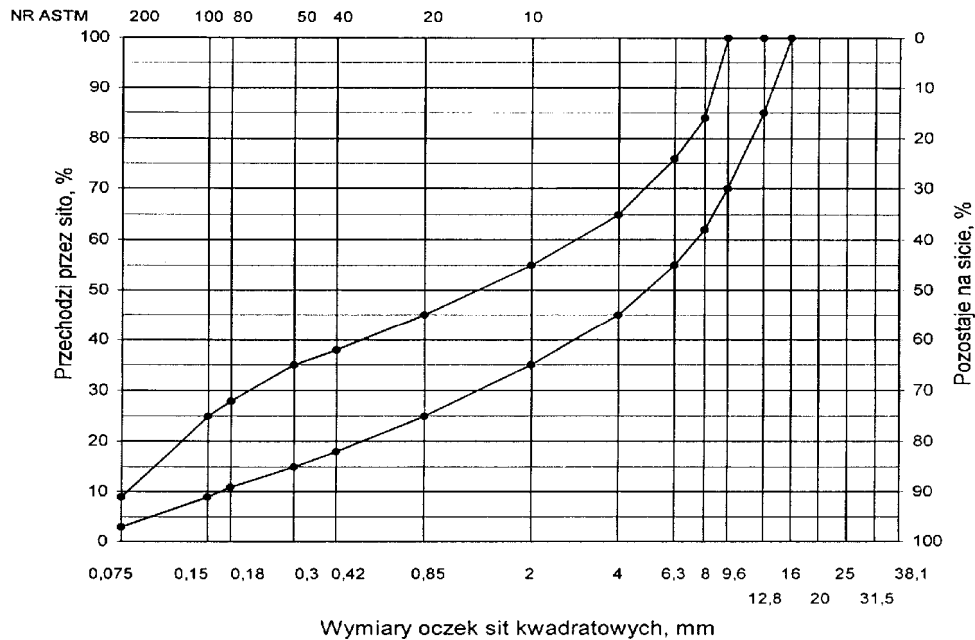
Rys. 10. Krzywe graniczne uziarnienia mieszanki mineralnej BA od 0 do 12,8 mm do warstwy wyrównawczej i wzmacniającej nawierzchni drogi o obciążeniu ruchem KR1 lub KR2
